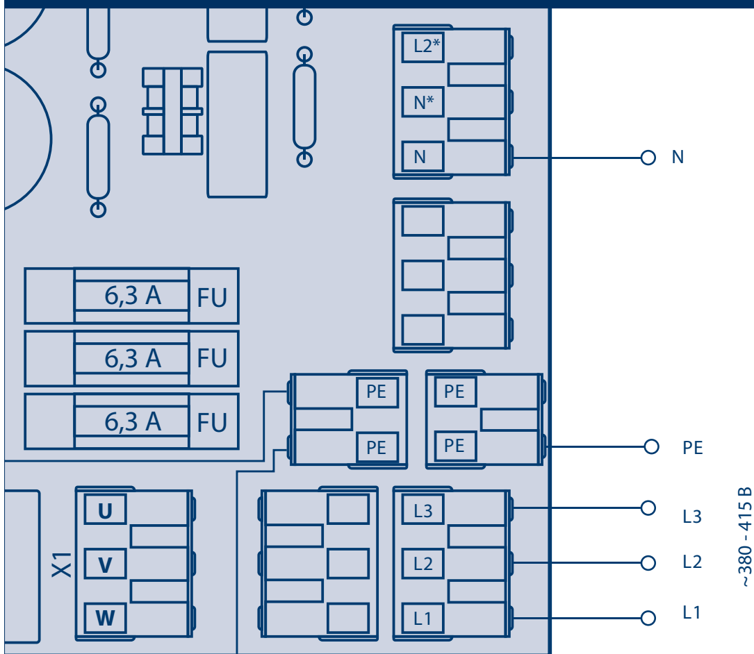
Рис. 5.2.1. Вид А. Подключение источника питания
