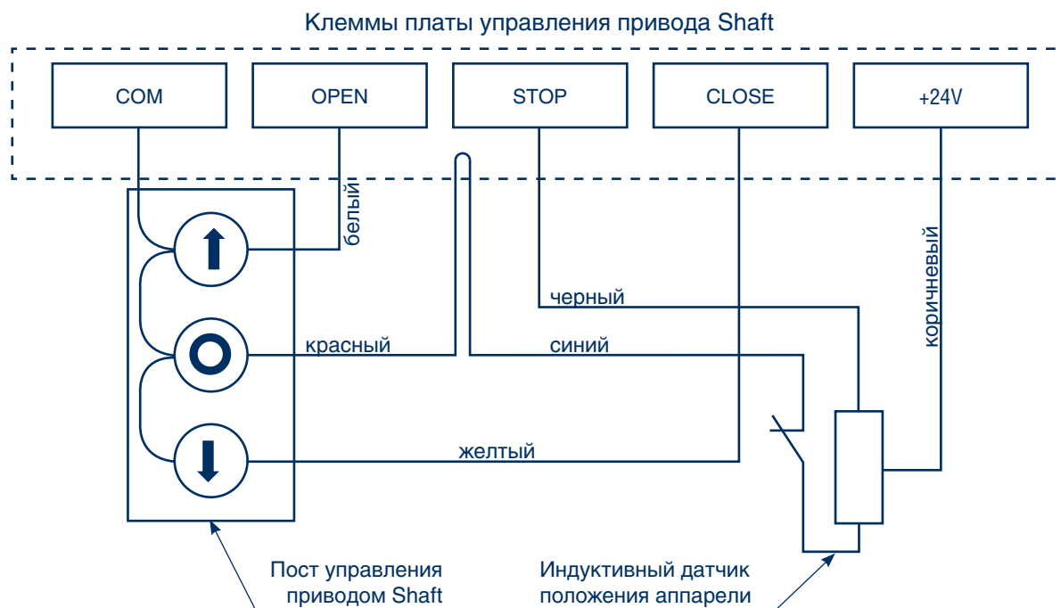
Рис. 5.5. Схема подключения индуктивного датчика положения аппарата для блока DCUH-2*
