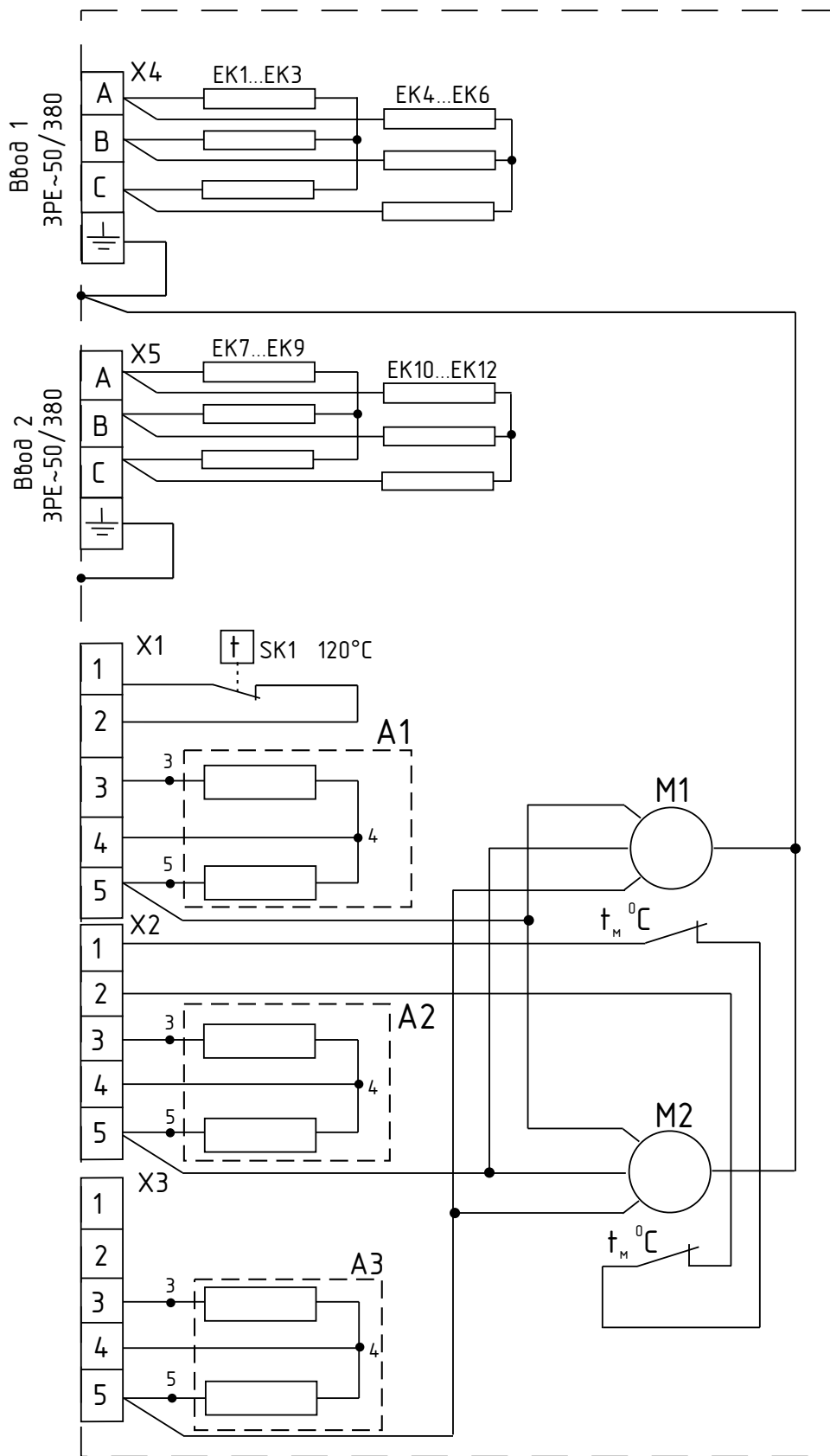
Рисунок 3. Электрическая схема занавесы КЭВ-24П7011Е, КЭВ-36П7011Е
