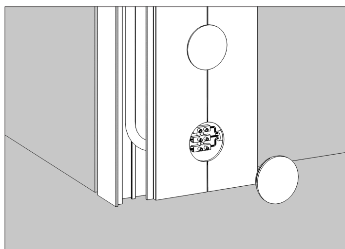
Установите клеммную колодку с соединенными проводами в монтажное отверстие. Отверстие закройте декоративной заглушкой.
