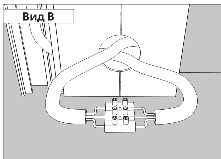
С помощью клеммной колодки соедините кабель обогрева рамы и кабель питания.
