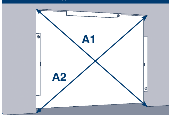
Рис. 7.1.2. Разность диагоналей
