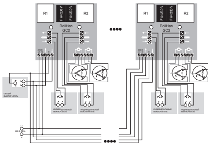
Рис. 3. Схема соединений блоков GC2
