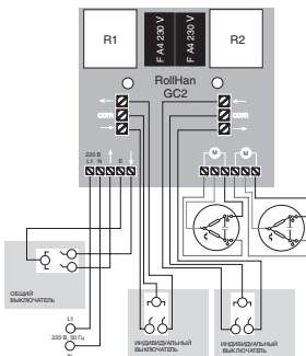
Рис. 2. Схема подключения группового управления GC2
