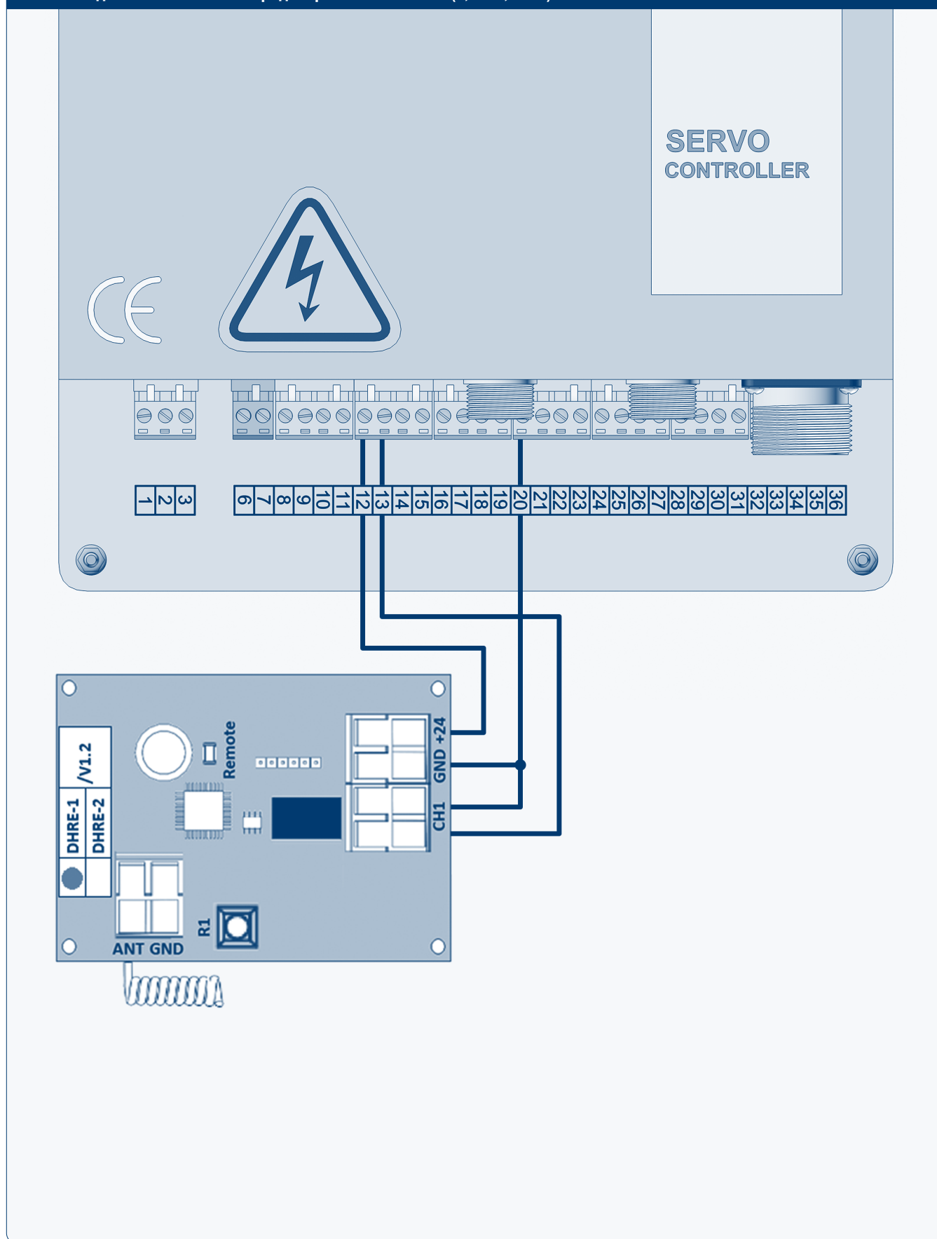
Рис. 17. Подключение внешнего радиоприемника DHRE-1 (1,5 и 2,2 кВт)
